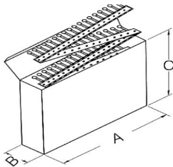
折叠式 Taping/Ammo
