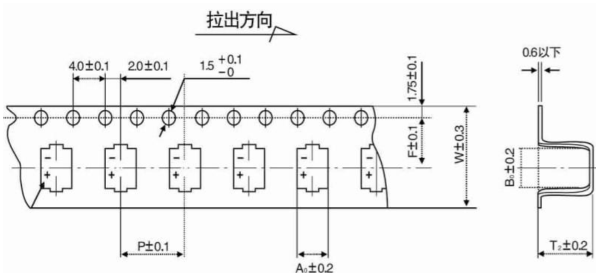
Fig.1 (Ø4 ~ Ø10)
